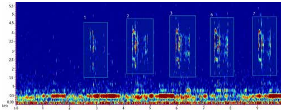
Abb. 5 | Spektrogramm eines Rebhahnrufes. Die x-Achse zeigt die Zeit in Sekunden und die y-Achse die durch die von 16:00 bis 20:20 Uhr (UTC) per Audiorekorder aufgenommene Frequenz (kHz). Im sogenannten Spektrogramm sind Dauer, Lautstärke (Farbgebung oder Farbtintensität) und Tonhöhe (Frequenzbereich) der einzelnen Rufelemente zu erkennen. Zwischen Sekunde 2,5 und 10 gibt es jeweils kurze Zeitfenster (kürzer als eine Sekunde), in denen der Balzruf des Rebhahns erfolgt. Die gewonnenen Aufnahmen wurden mittels einer angepassten Version des KNN BirdNET ausgewertet und aufgrund Ihrer Spektrogramme (Abb. 2) evaluiert.
